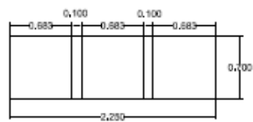
planta/sezione
