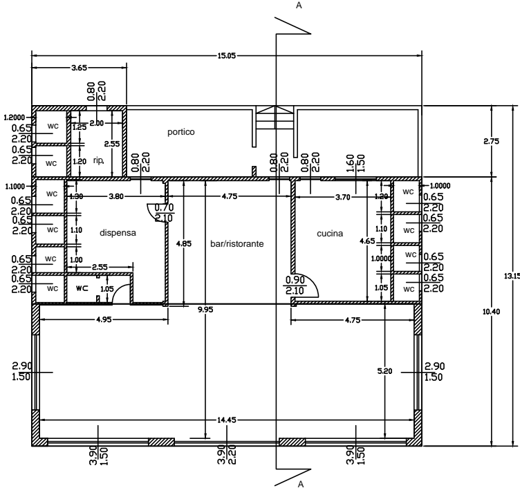
PIANTA PIANO TERRA stato di fatto
