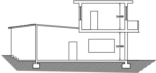
SEZIONE A-A stato di fatto
